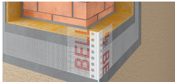
BP23 S KĄTOWNIK PVC Z GRZBIETEM 4mm Z SIATKĄ
