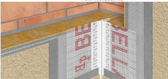
BP16 V LISTWA PVC DYLATACYJNA TYPU „V” - KĄTOWA Z SIATKĄ
