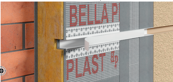
BP11 H2 NS LISTWA PVC DO BONIOWANIA ZAMKNIĘTA Z ELEMENTEM TRACONYM I Z SIATKĄ, 20x20mm
