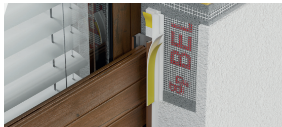
BP13 R LISTWA DYLATACYJNA DO PROWADNIC ROLET W SYSTEMACH ROLET OKIENNYCH ZEWNĘTRZNYCH
