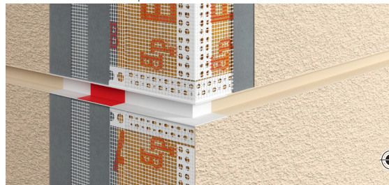
BP11 H3 R ZEW KĄTOWNIKI PVC ZEWNĘTRZNE DO BONI
